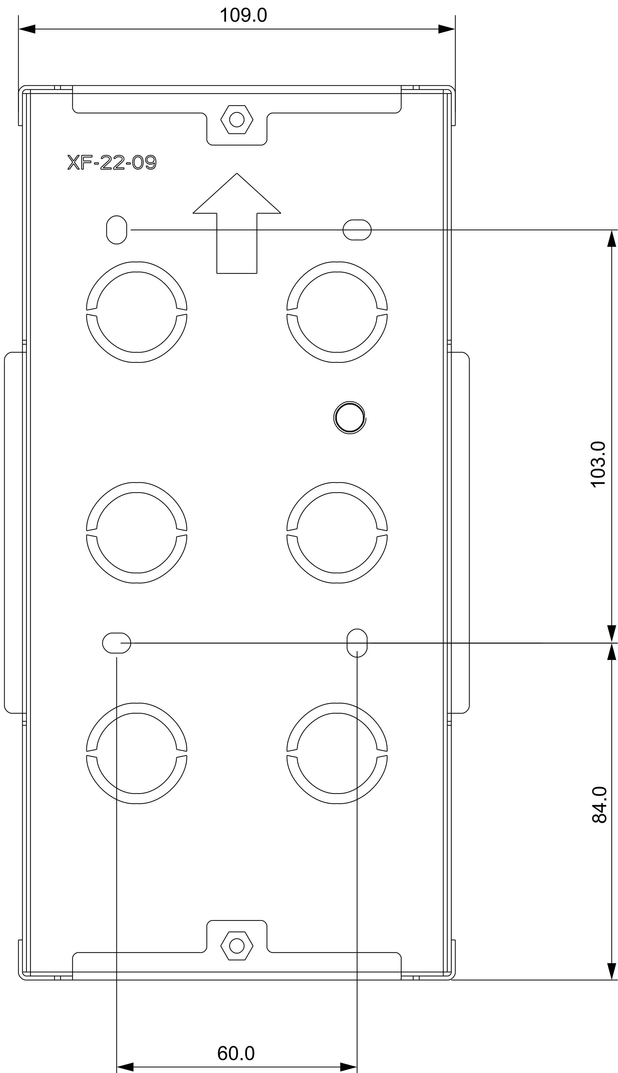
1 主视图
