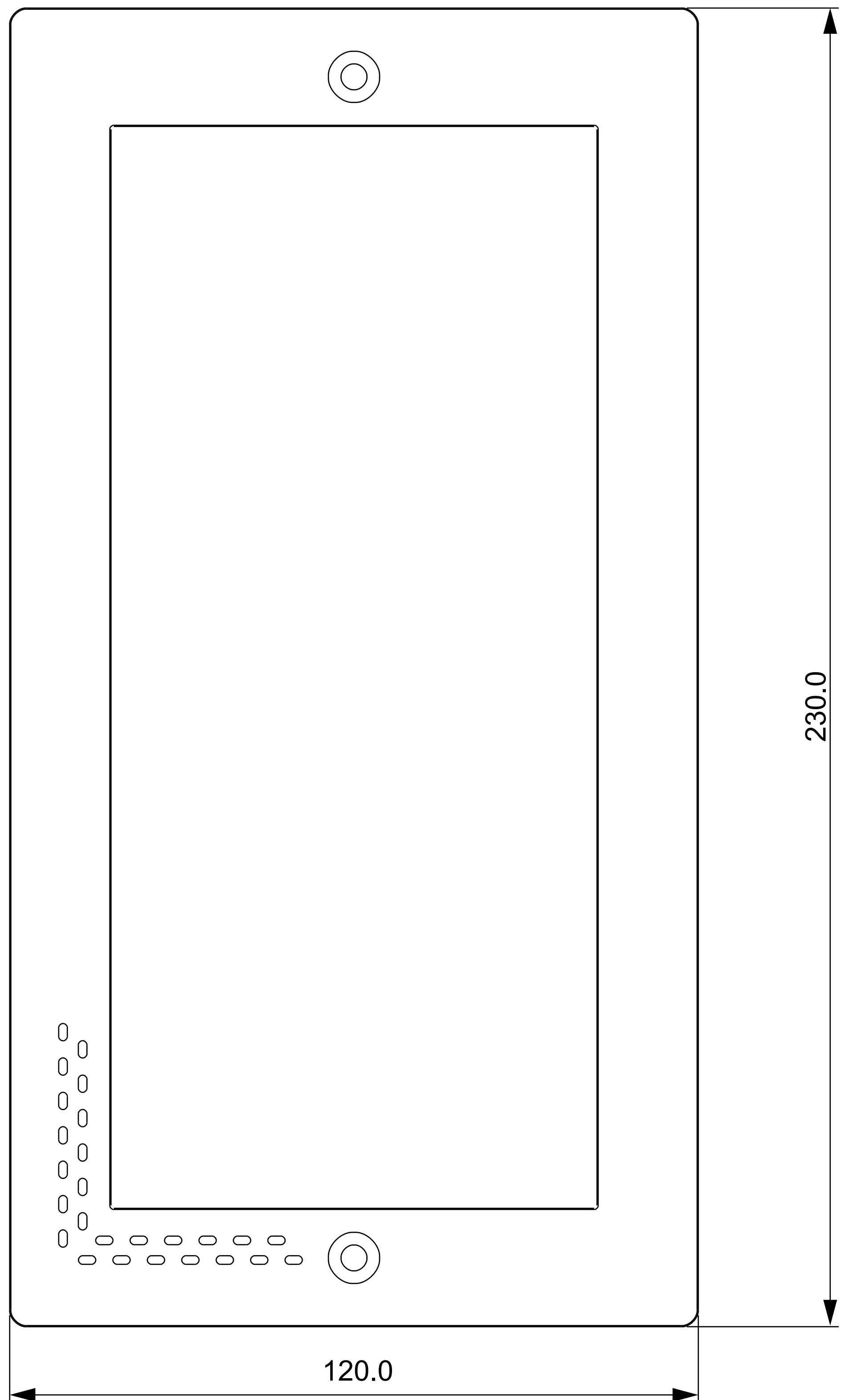
① 主视图
