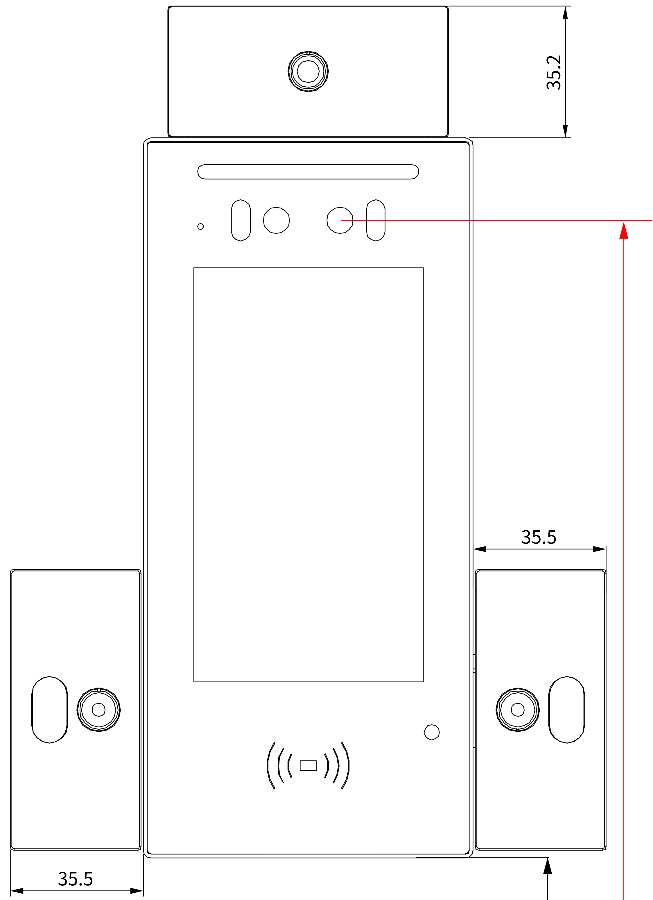
① 带温度测量模块的对讲机面板正视图
