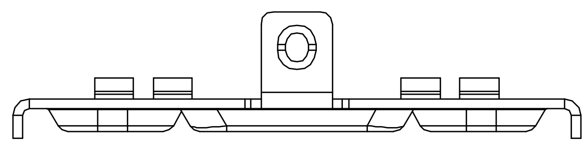
6 仰视图
