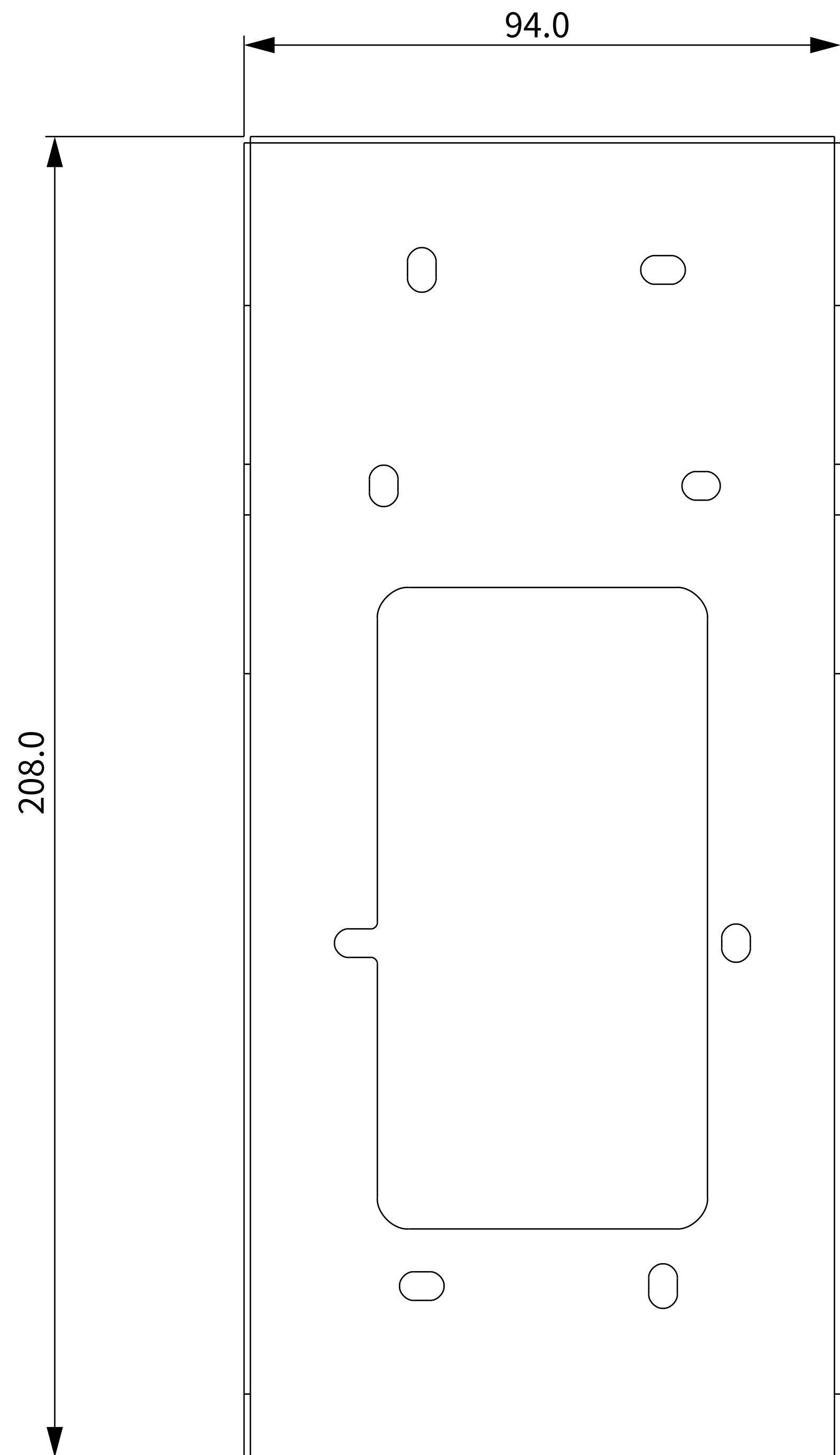
① 正视图
