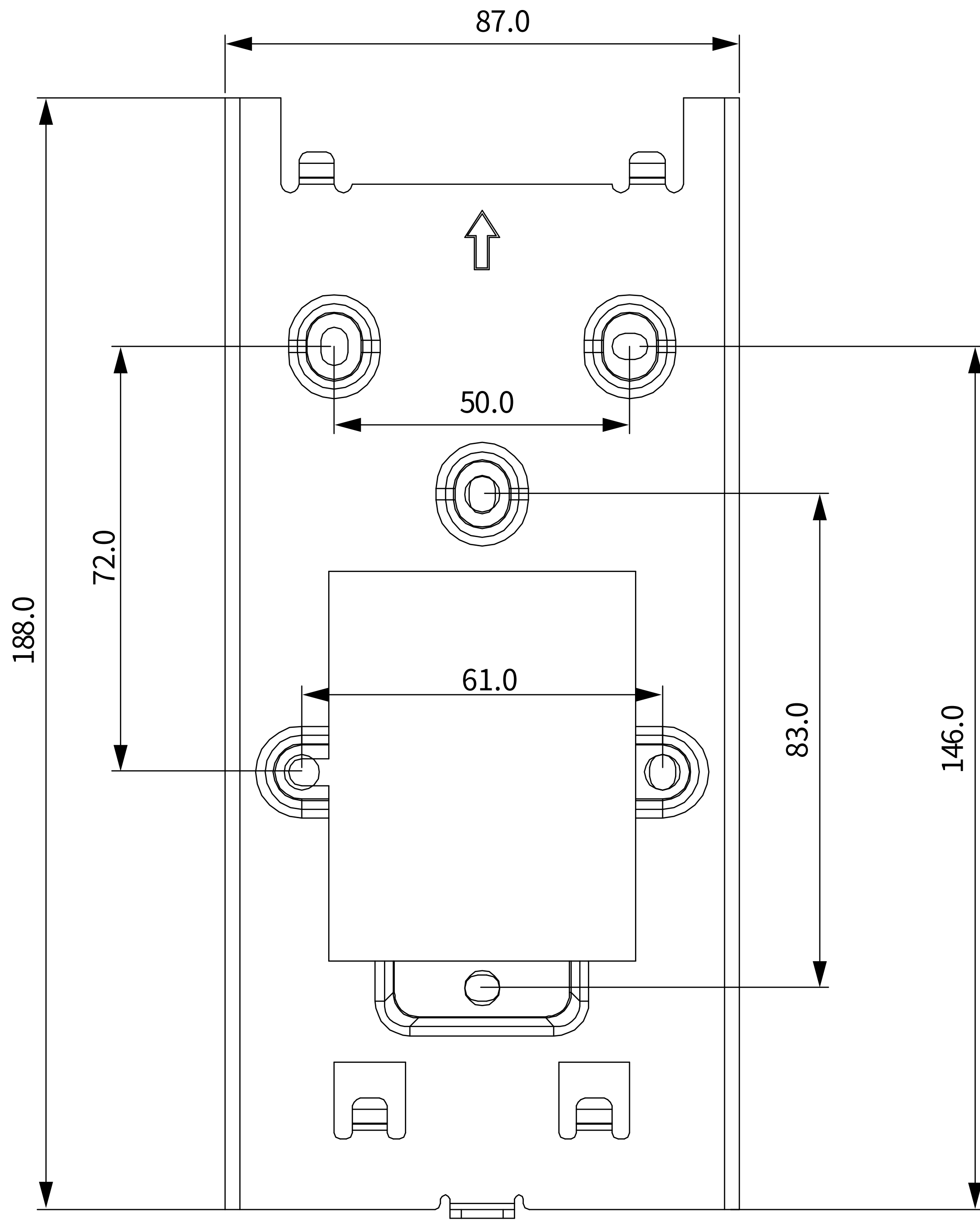
1 正视图
